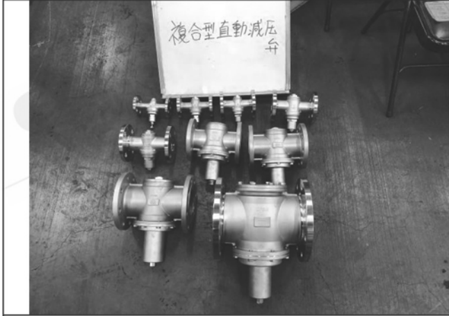
照片 A：測試樣品外觀 複合型-直動減壓閥(法蘭)
