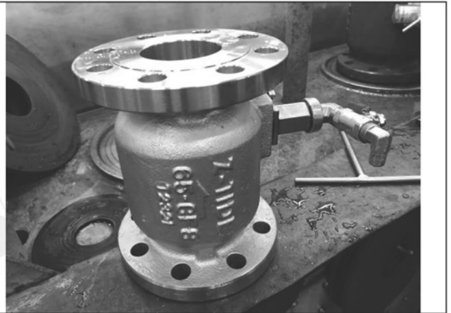
照片 B：測試樣品外觀 (DN65)BFF-65
