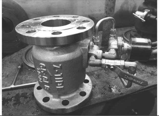
照片 B：測試樣品外觀 (DN65)BFE-65
