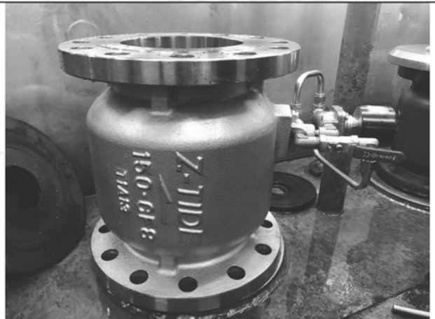
照片 F：測試樣品外觀 (DN150)BFE-150
