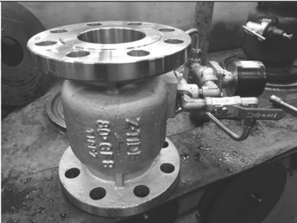
照片 C：測試樣品外觀 (DN80)BFE-80
