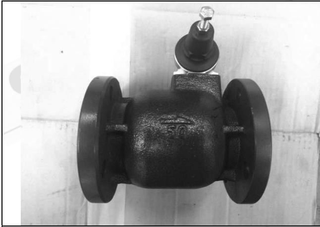
照片 A：測試樣品外觀 (DN50)BFR-50
